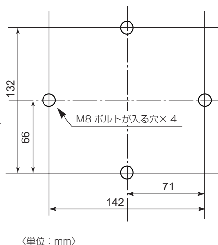
〈つりボルト取り付け穴寸法〉
