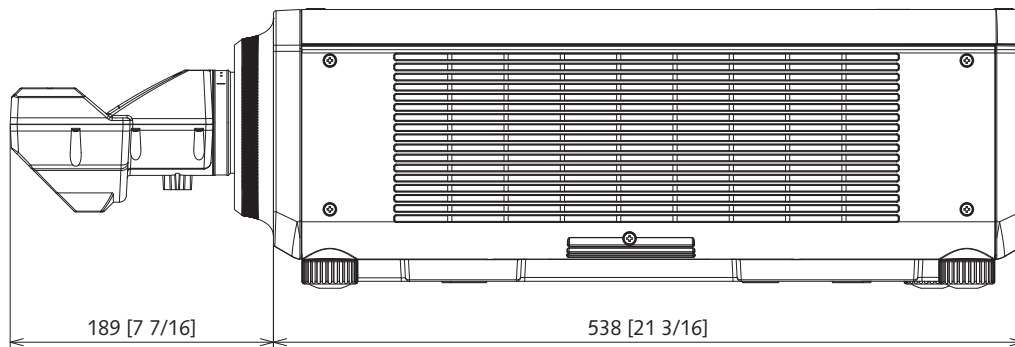
ET-DLE035+PT-RCQ10/PT-RCQ80/PT-RZ120/PT-RZ990/PT-RZ890/PT-RZ790/ PT-RZ690/PT-RZ970/PT-RW930/PT-RX110/PT-RZ870/PT-RZ770/ PT-RW730/PT-RZ660/PT-RW620
