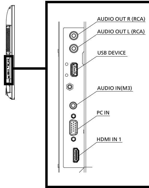
端子部拡大図 b
