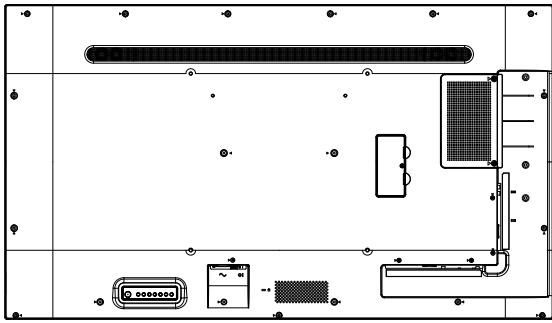
背面視
