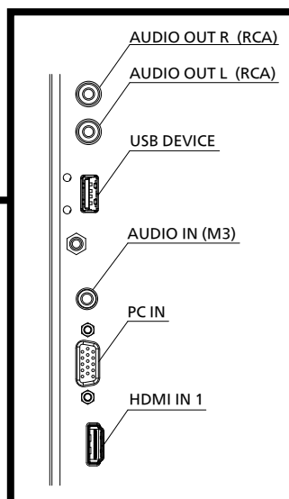
端子部拡大図 b
