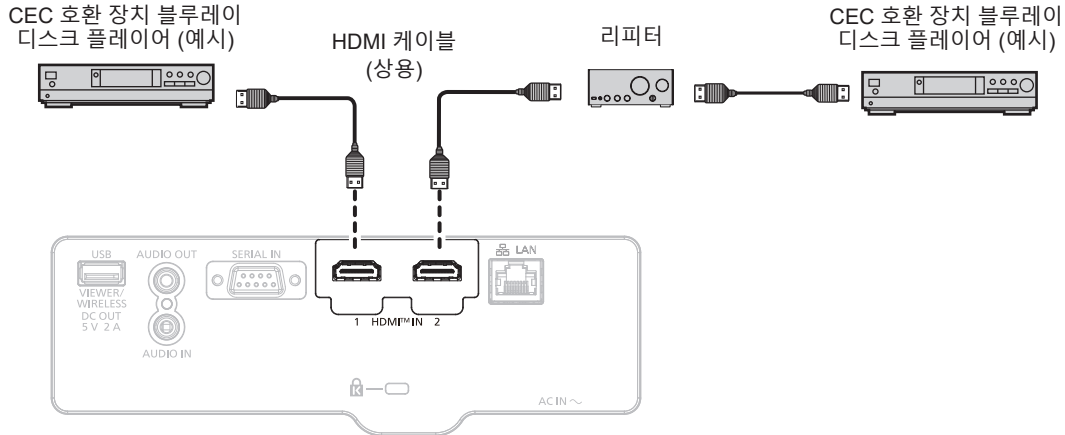
CEC 호환 장치와의 연결 예
