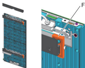
Vista posteriore del modulo mobiletto
