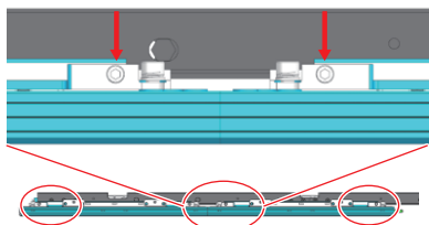
Vite di regolazione dell'asse Y
