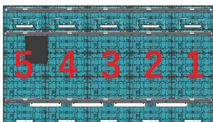
Rückansicht Cabinet-Modul
