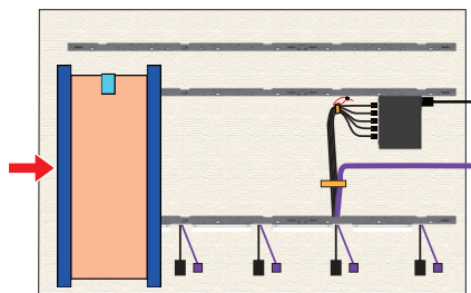
Rückansicht Cabinet-Modul
