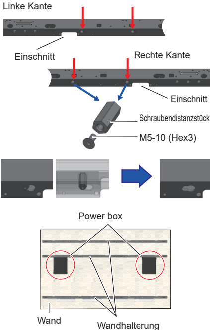
Wandhalterung
