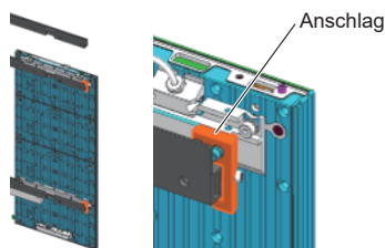
Rückansicht Cabinet-Modul
