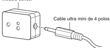
Módulo sensor
