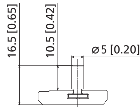
フレーム組付け状態 Frame assembly condition
