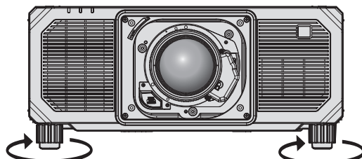
Plage de réglage maximale Pieds réglables : 20 mm (25/32") chacun
