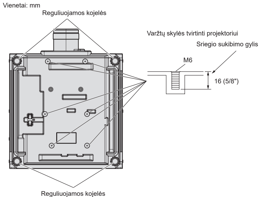
Varžtų skylių vietos tvirtinti projektoriui ir reguliuojamoms kojelėms.
