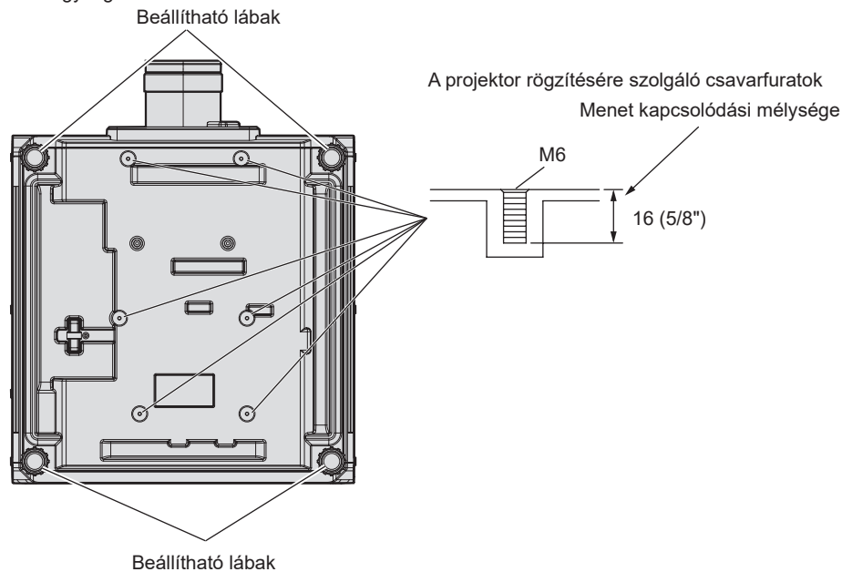
A projektor rögzítésére szolgáló menetes furatok és a beállítható lábak elhelyezkedése
