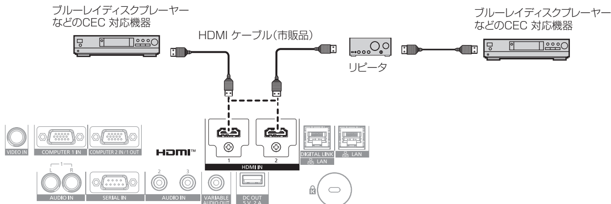
CEC 対応機器との接続（例）
