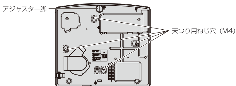
天つり用ねじ穴 (M4) とアジャスター脚の位置
