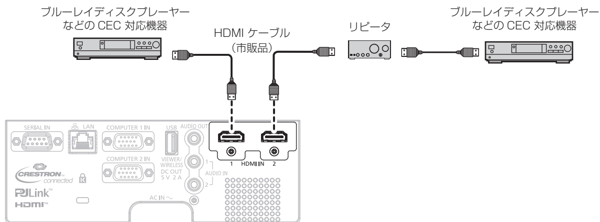
CEC 対応機器との接続（例）
