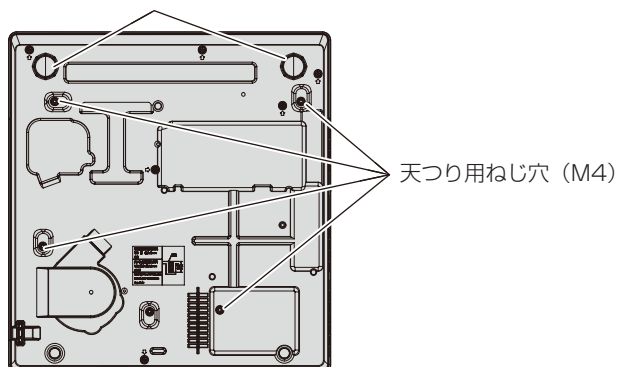
天つり用ねじ穴 (M4) とアジャスター脚の位置
