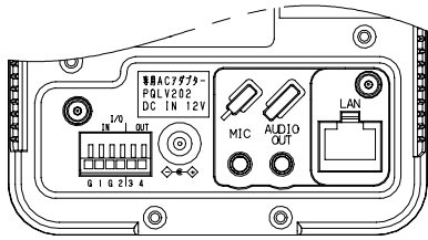
ケーブルカバー取り外し状態
