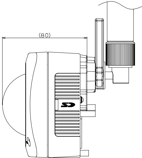
サンシェードを外した状態図
