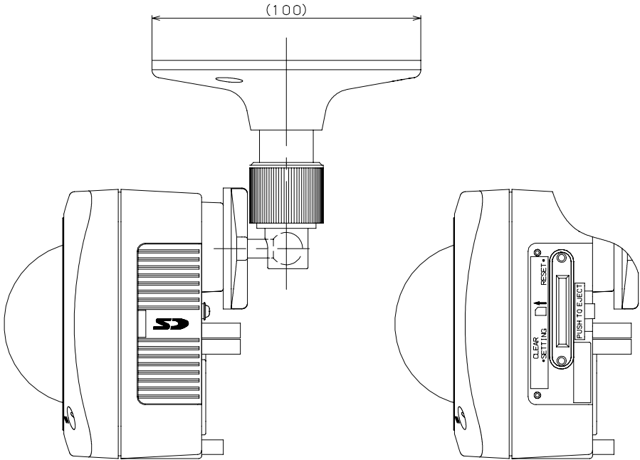
サンシェードを外した状態図
