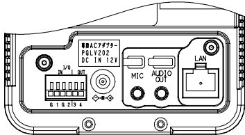
ケーブルカバー取り外し状態
